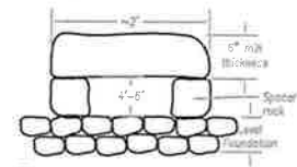
2A SIDE
