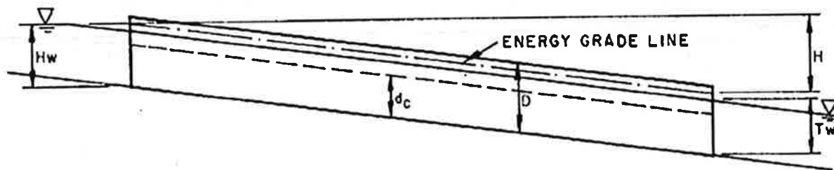
Figure 1000-8. Partially Full Conduit (UDFCD, 2016).
