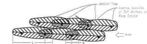
3 JUNIPER REVETMENT
