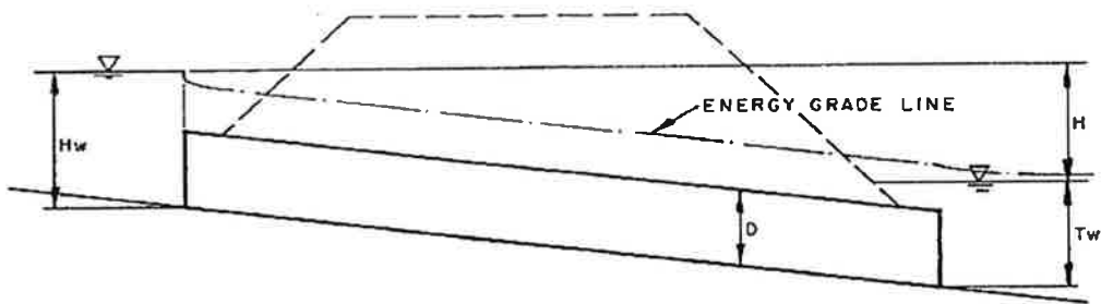
Figure 1000-9. Full Conduit (UDFCD, 2016).
