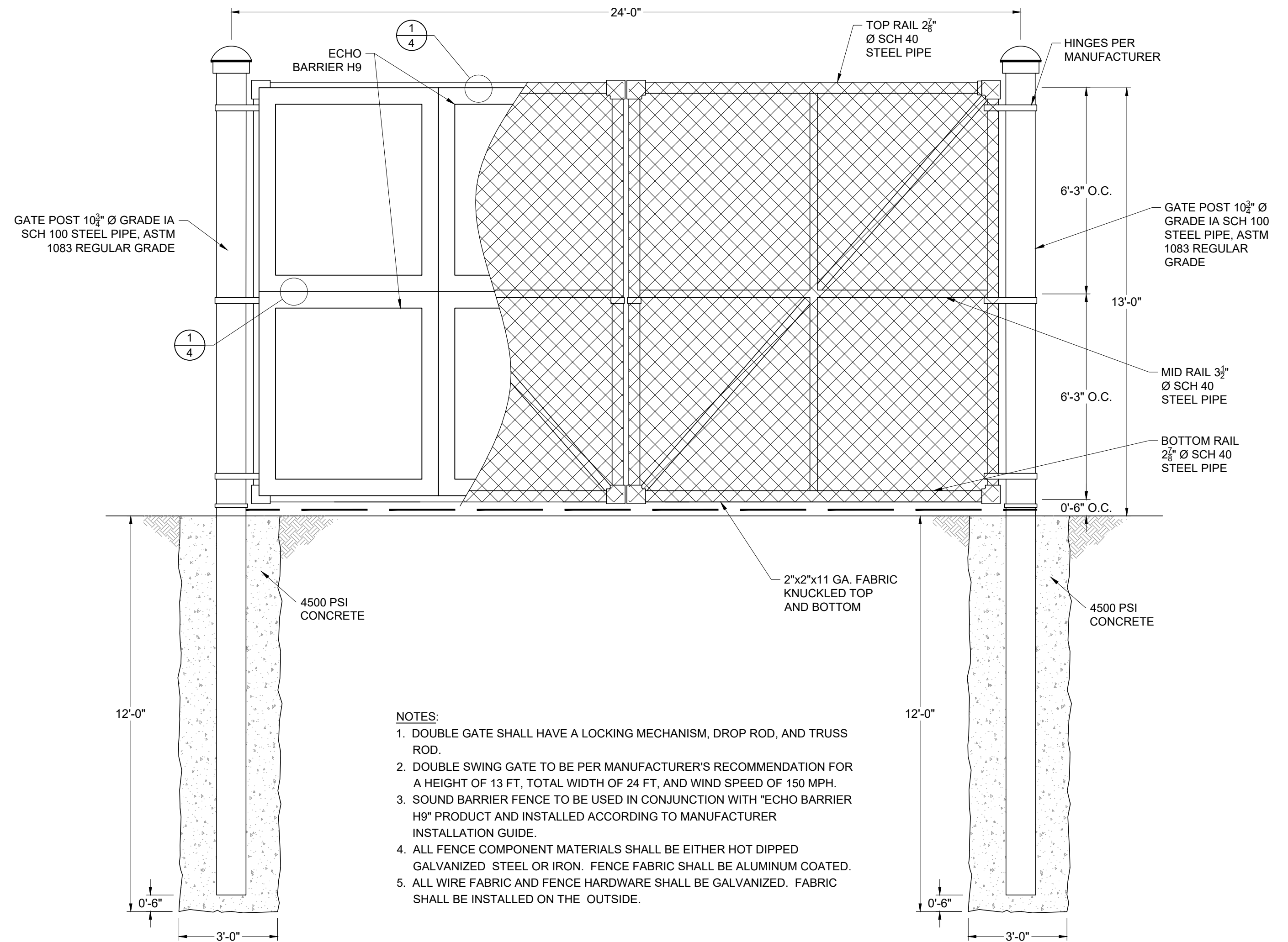
A GATE SECTION 4 SCALE: 3/8" = 1'-0"
